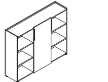
Contentore con anta scorrevole/ Cabinet with sliding door L 160 P 40 H 120
